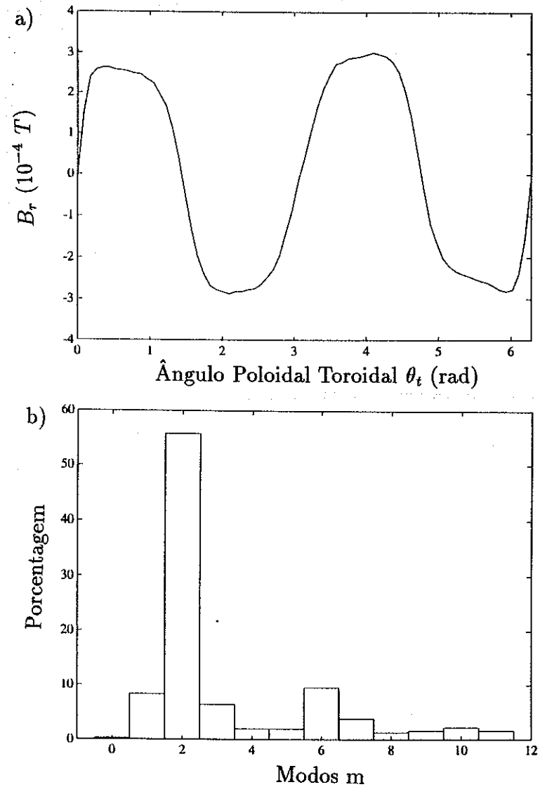
Fig. 17 - Perfil poloidal de B_r criado pela malha do CHR m/n = 2/1 em \rho_t = 7,73 cm (a) e sua composição de modos (b).
