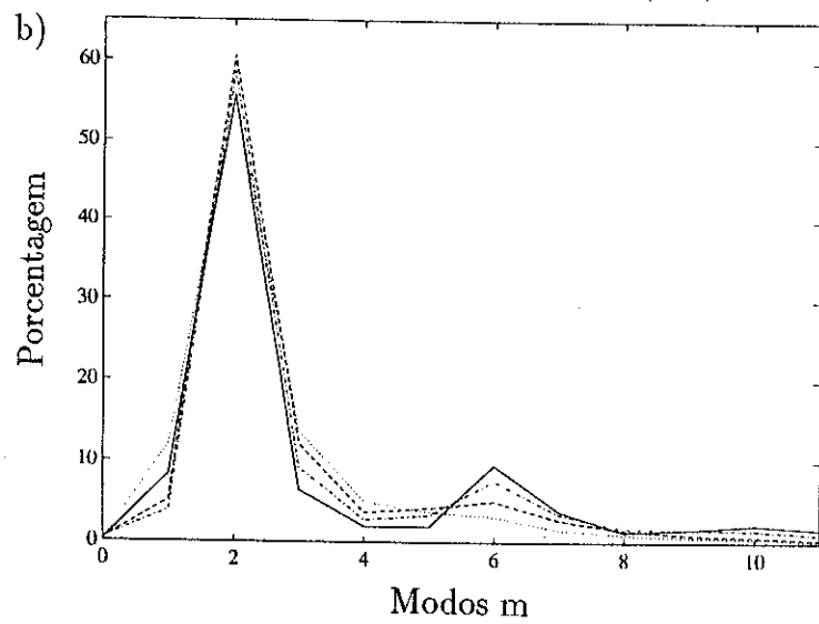
Fig. 18 - Gráfico conjunto dos perfis poloidais de B_r medidos nas 4 superfícies de \rho_t constante (a) e suas respectivas composições de modos (b) referentes ao CHR m/n = 2/1 .
