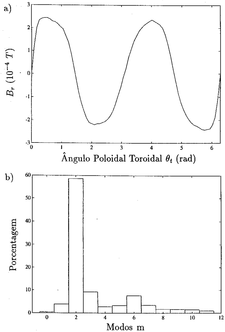
Fig. 16 - Perfil poloidal de B_r criado pela malha do CHR m/n = 2/1 em \rho_t = 7,0 cm (a) e sua composição de modos (b).
