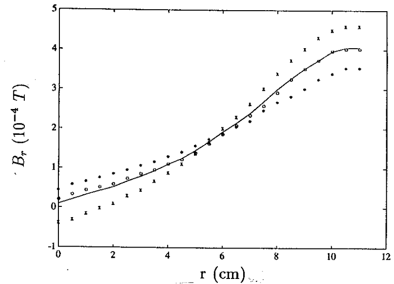
Fig. 13 - Perfil radial de B_r criado pelo enrolamento do CHR m/n = 4/1 , medido nas posições \theta = 65^\circ (*), \theta = 145^\circ (x) e \theta = 330^\circ (o). A curva contínua representa a média dos valores obtidos.
