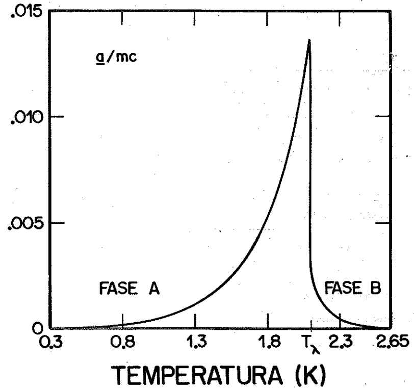
FIG. 7 - "NÚMERO DE SÓLITONS": g/mc .
