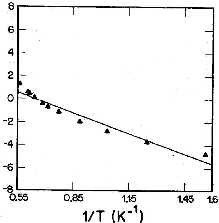
FIG. 11 - LOGARITMO DO CALOR ESPECÍFICO (▲) VS. O INVERSO DA TEMPERATURA, NO INTERVALO DE 0,6K - 1,8K. A RETA CONTÍNUA DÁ A DERIVADA MÉDIA, OU O GAP MÉDIO (-6,2K).
