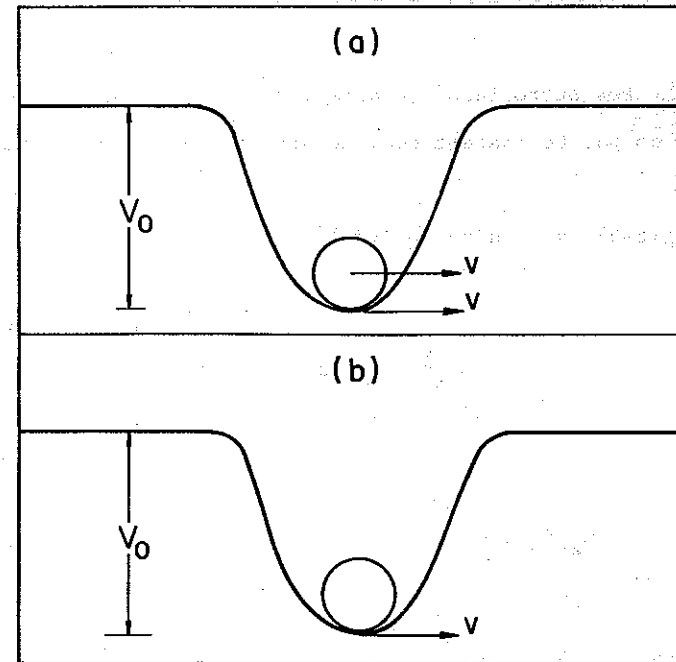
FIG. (2) - CONFIGURAÇÕES CLÁSSICAS ANÁLOGAS : (a) A PARTÍCULA SE MOVE JUNTO COM O POTENCIAL - SITUAÇÃO ANÁLOGA AO ESTADO LIGADO \psi_0 ; (b) A PARTÍCULA, NO INSTANTE t=0 , ESTÁ EM REPOUSO COM RELAÇÃO AO LABORATÓRIO - SITUAÇÃO ANÁLOGA AO PACOTE INSTANTÂNEO f_0 .
