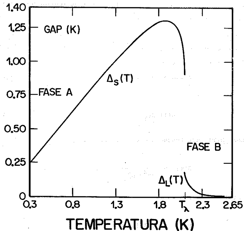
FIG. 5 - TRAJETÓRIAS DO GAP - FASE A: \Delta_S(T) ; FASE B: \Delta_L(T) .
