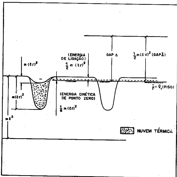
FIG. (3) - DISPOSIÇÃO DOS NÍVEIS DE ENERGIA DO PROBLEMA.
