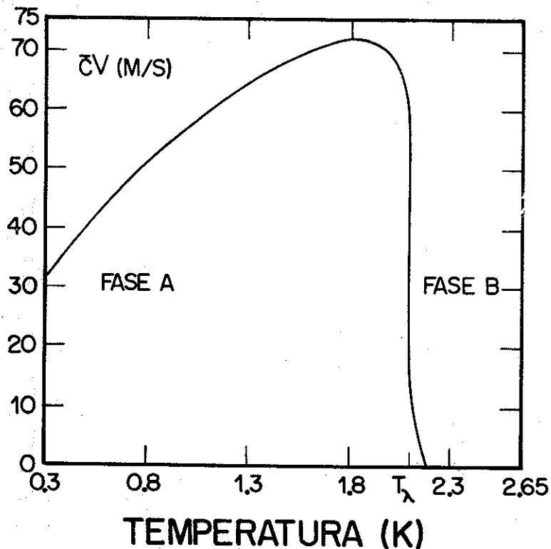
FIG. 9- VELOCIDADE DOS SÓLITONS EM M/S.
