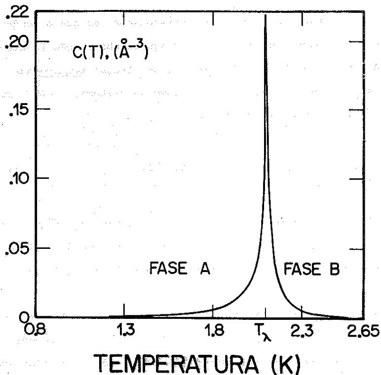
FIG. 10 - CALOR ESPECÍFICO DO SISTEMA DE SÓLITONS.
