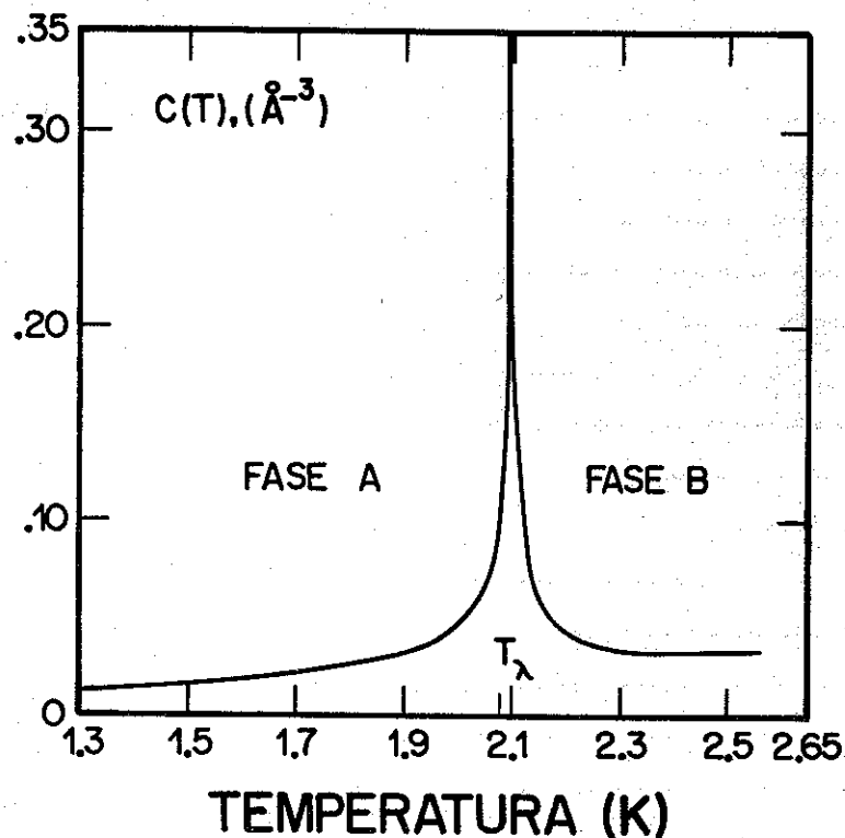
FIG. 1- CALOR ESPECÍFICO DO SISTEMA DE SÓLITONS SOMADO AO CALOR ESPECÍFICO DO FLUIDO NORMAL.
