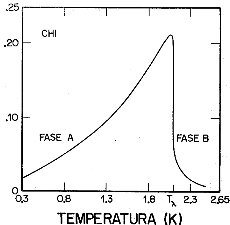
FIG. 8 - ÍNDICE DE PROFUNDIDADE.
