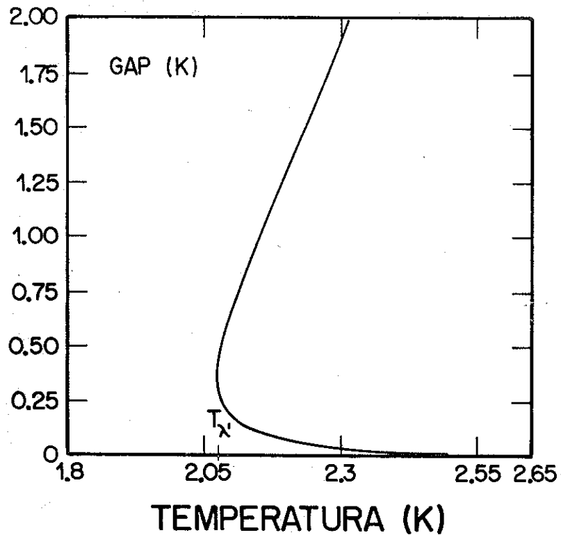
FIG. 4 - REGIÃO DE SATURAÇÃO NO PLANO \Delta \times T .
